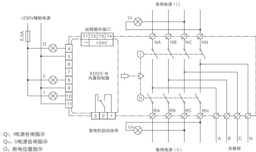
XDQ3-B型ATS开关应用接线图（4P）
