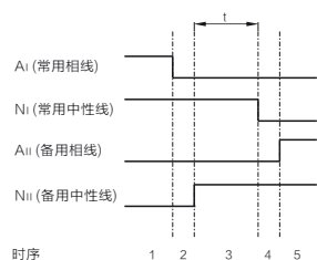
常转备时序图
