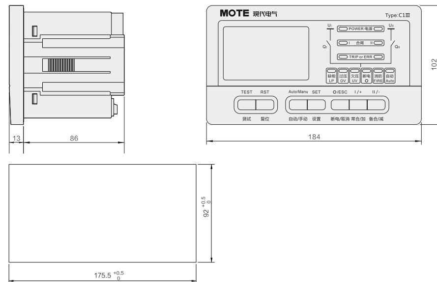
C1型面板开孔尺寸
