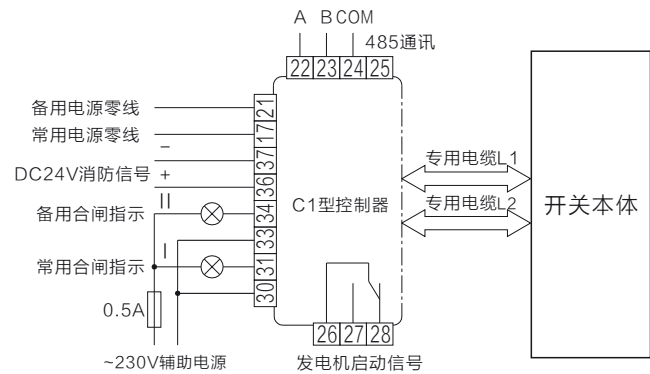
XDQ3-C1型接线图
