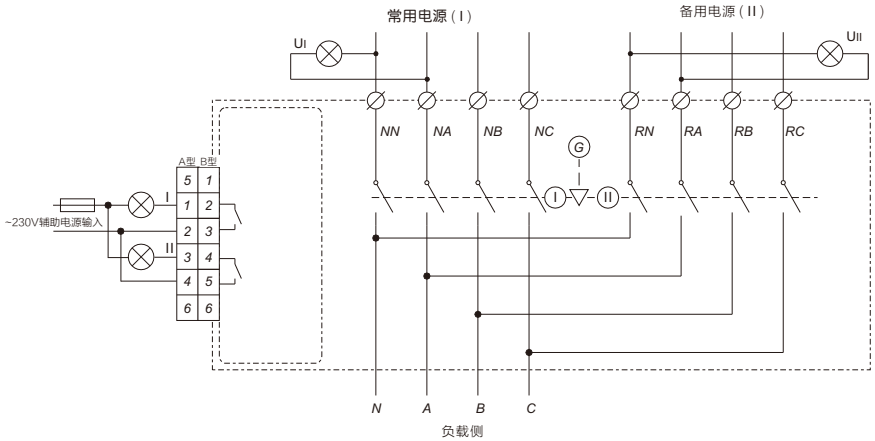
A、B型控制器应用接线图（4P）
