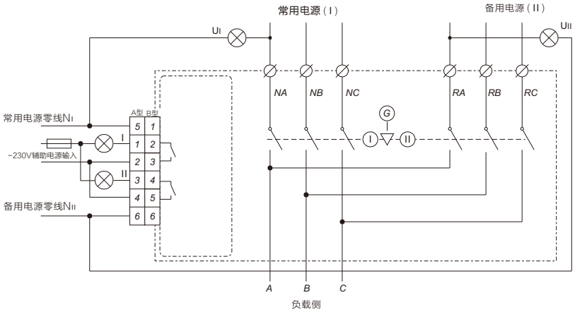
A、B型控制器应用接线图（3P）
